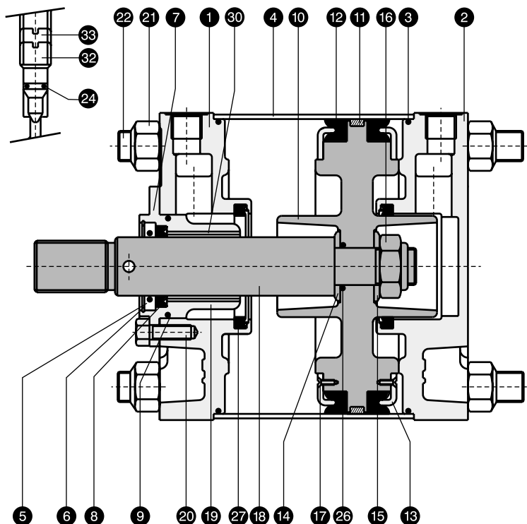
Ø 8", 10", 12" & 14" Cylinder
